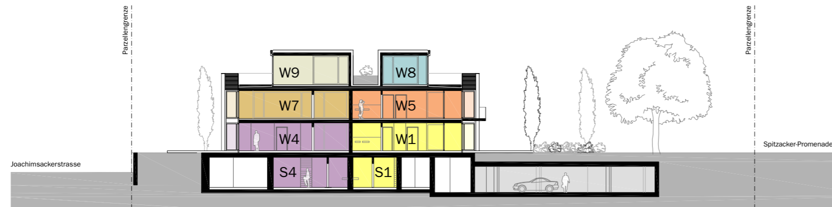
Schnitt B-B
