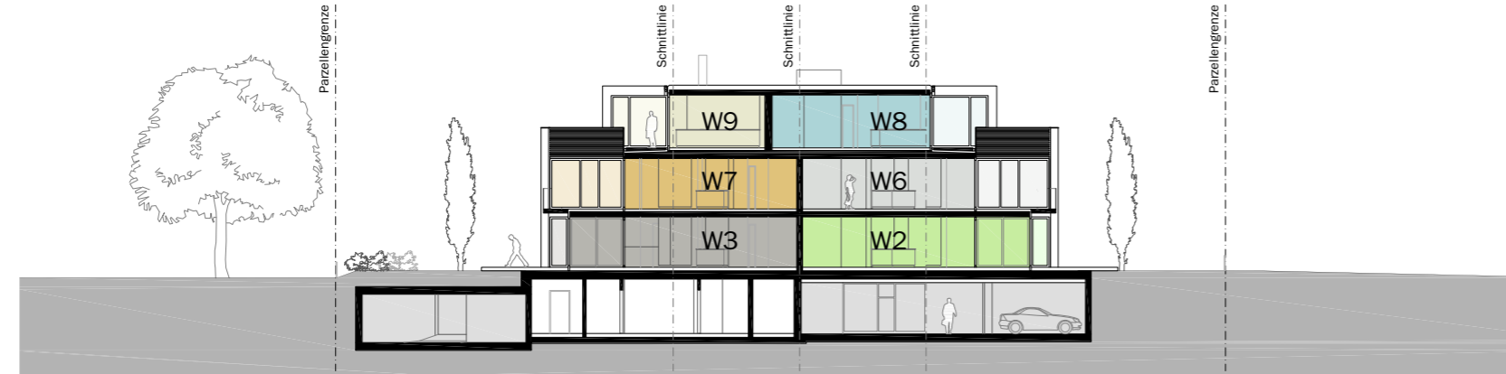
Schnitt A-A
